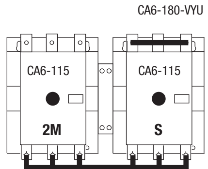
CA6-180-VLHB
